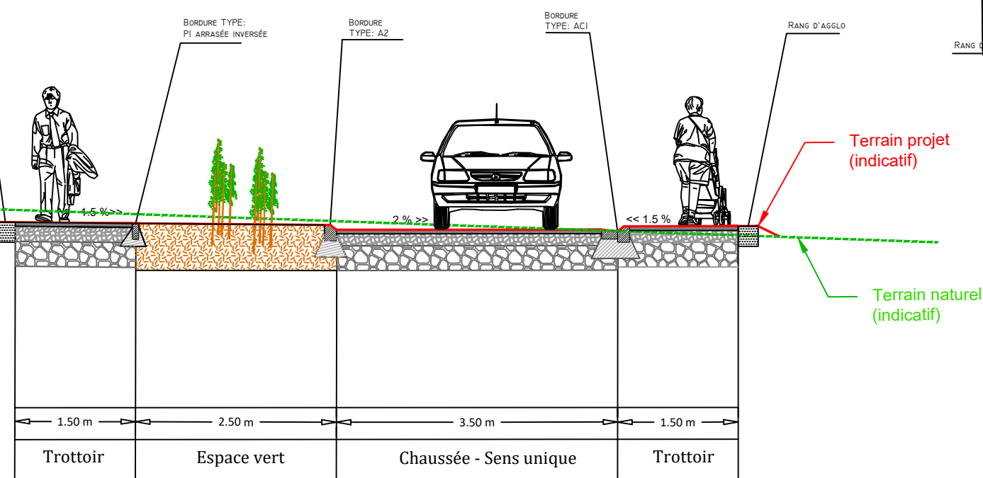
Coupe Voirie Type - BB' Schéma de principe Echelle 1/75 ème
