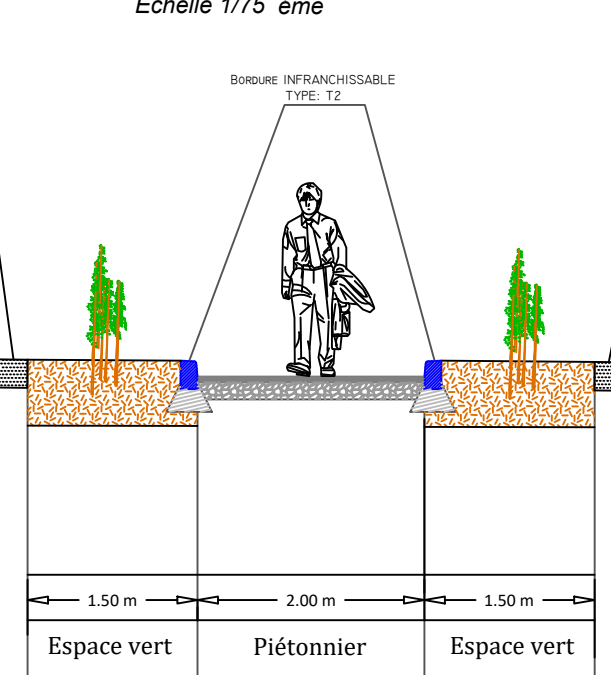
Coupe Voirie Type - CC' Schéma de principe Echelle 1/75 ème
