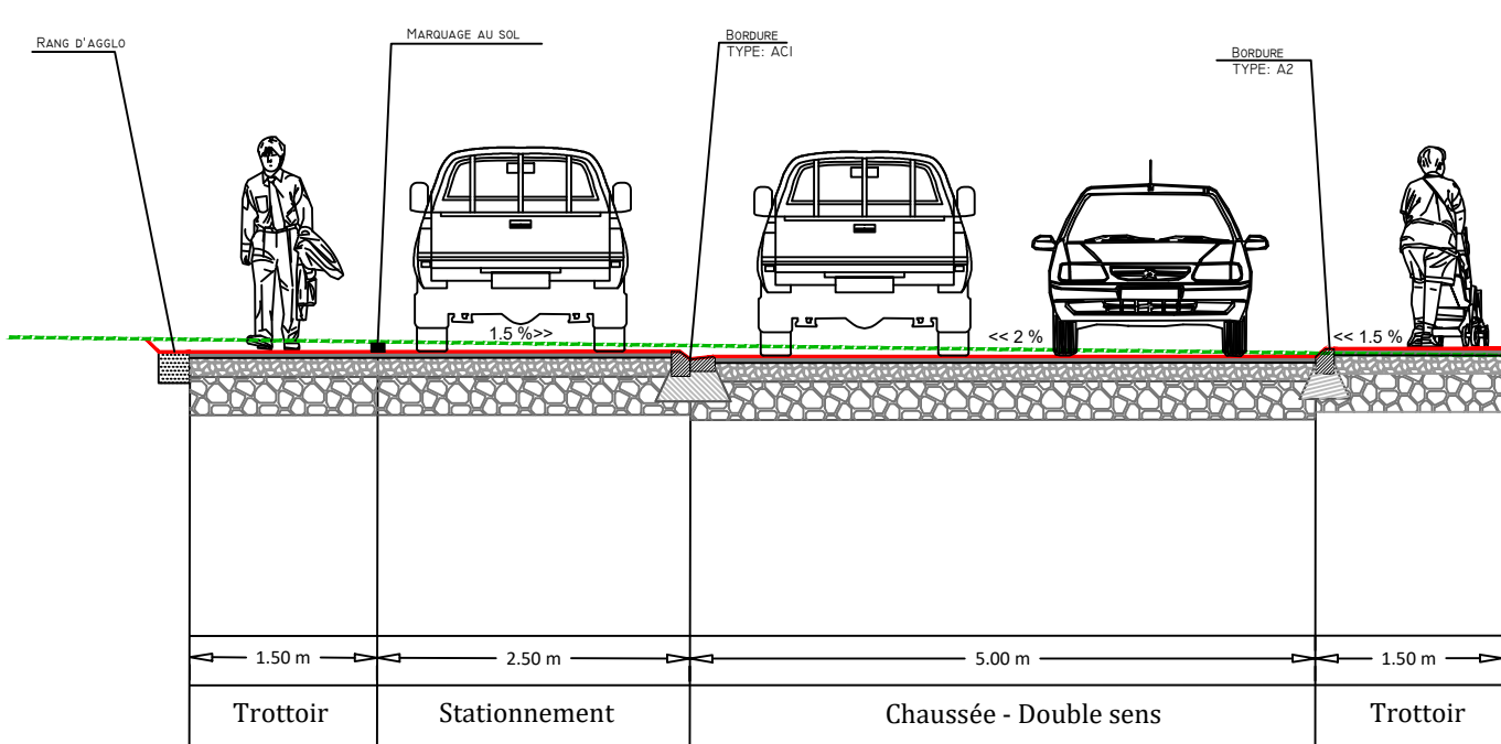
Coupe Voirie Type - AA' Schéma de principe Echelle 1/75 ème
