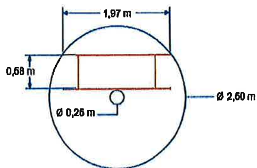
Figure 5 - Schéma d'un escalier hélicoïdal
