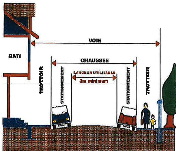
Figure 1 - Caractéristique d'une voie utilisable par les engins de secours (voies-engins)
