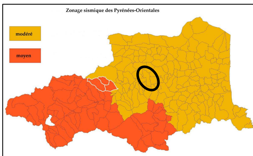
Figure 3 : Zones soumises au risque de mouvement de terrain des Pyrénées-Orientales
