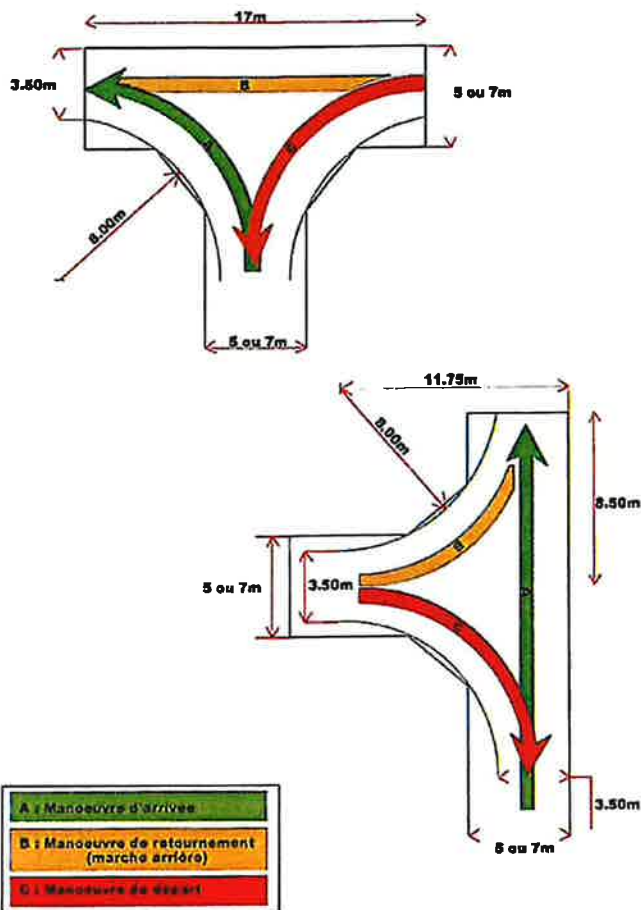
Figure 2 - Principe de retournement de type « raquette »
