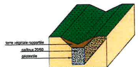
noue avec massif drainant
