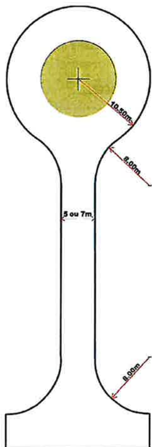
Figure 2 - Principe de retournement de type « raquette »
