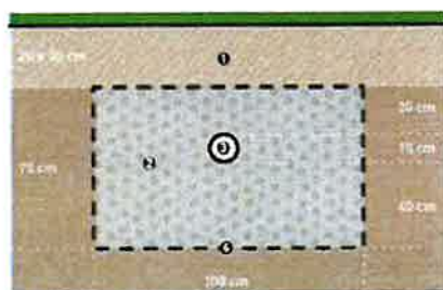
Tranchée filtrante
