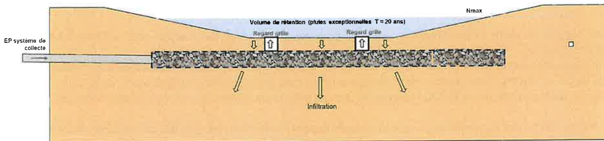
Figure - Principe de fonctionnement du bassin d'infiltration (coupe11')
