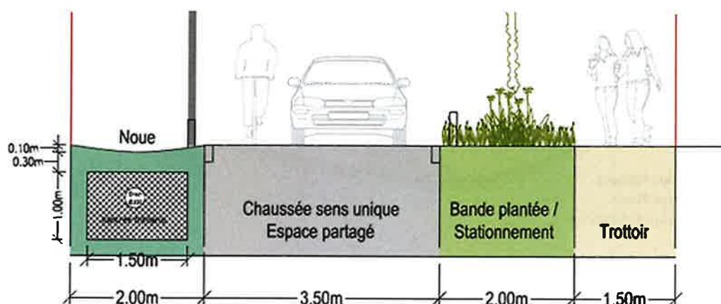
Principe de fonctionnement d'une noue drainée pour la gestion des pluies en domaine public
