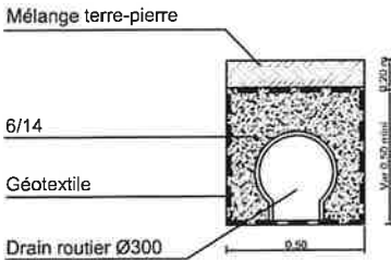
Coupe de la Tranchée de ressuyage Echelle : 1/10
