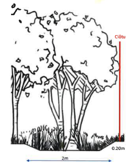
Schéma type d'une noue plantée
