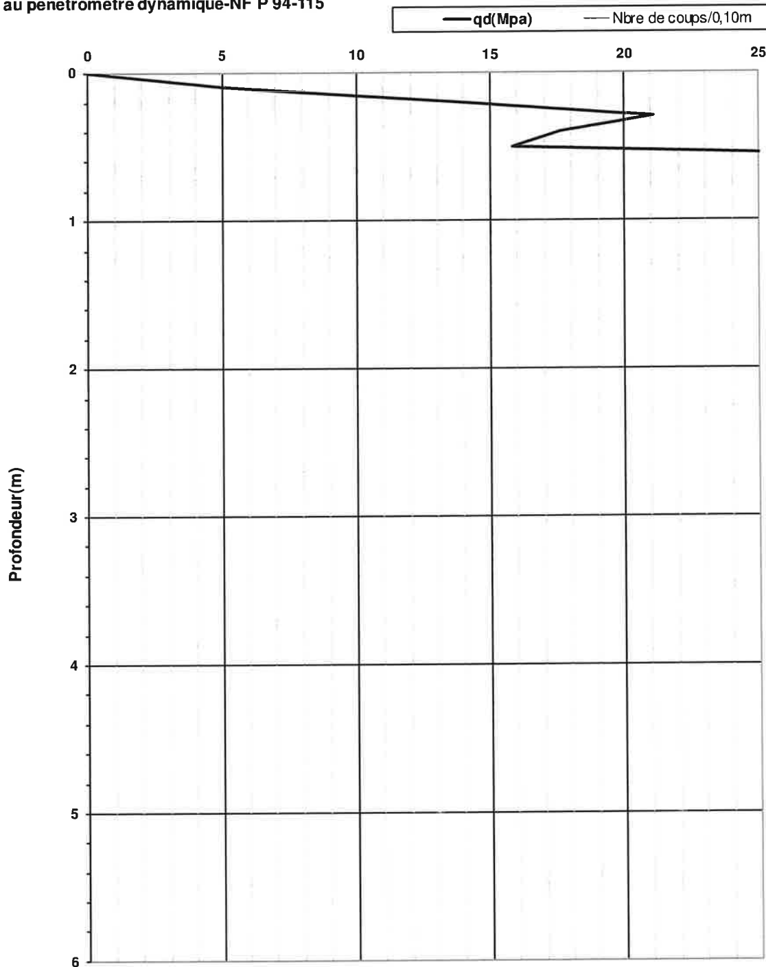
Sondage au pénétromètre dynamique-NF P 94-115
