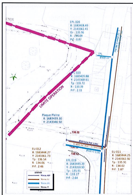
Figure 13 : Plan de recollement matérialisant les réseaux en attente à l'entrée du lotissement
