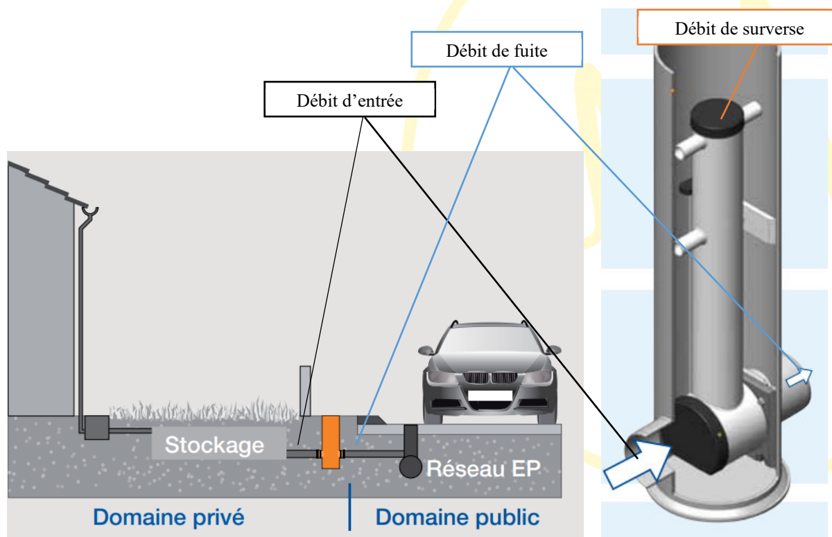
Schéma type d'un ouvrage de régulation – Modèle pris chez Wavin : Tabourets Corso 315
