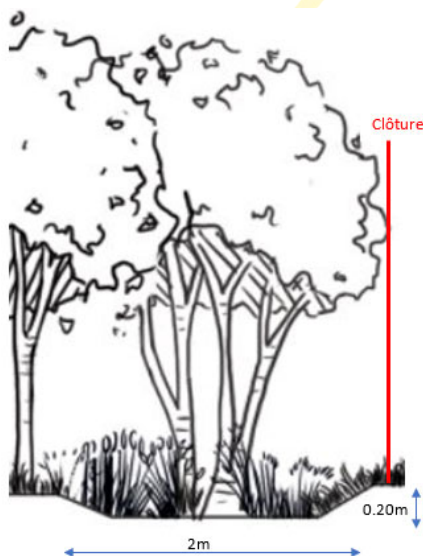
Schéma type d'une noue plantée
