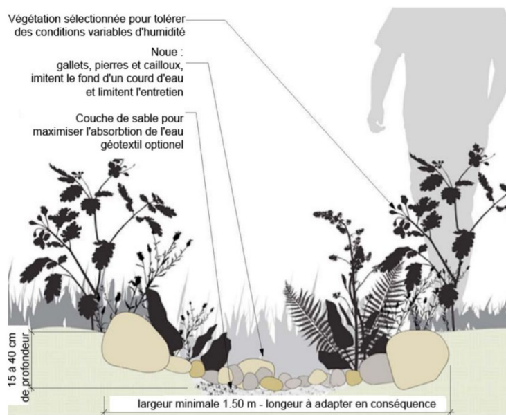
Schéma type d'un jardin de pluie
